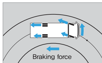
전자식 제동력 분배 시스템(EBD)
